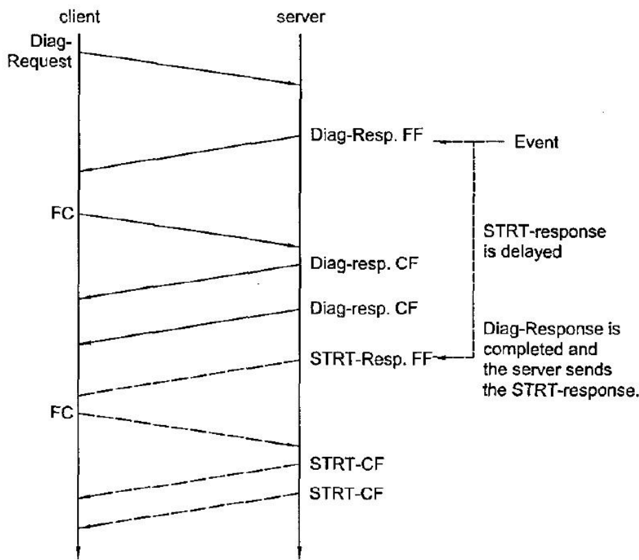
图 17——在一条信息处理过程中事件发生
