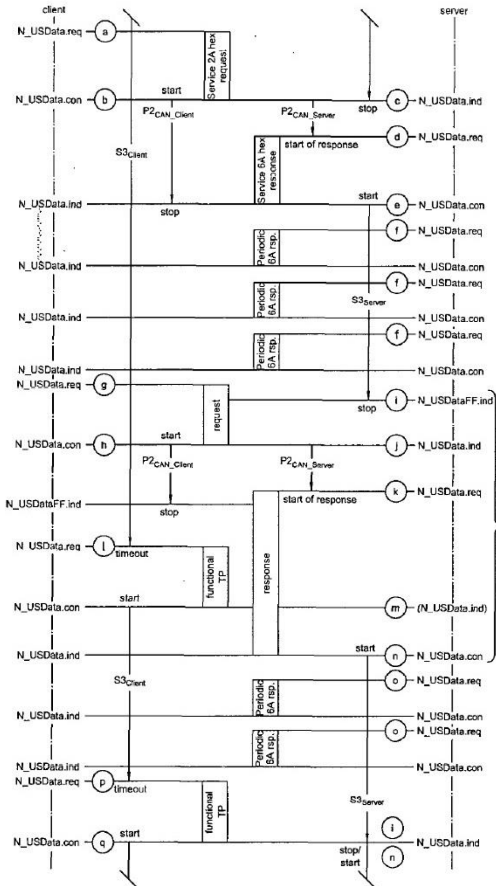
图 18——应答信息类型#1 的处理
